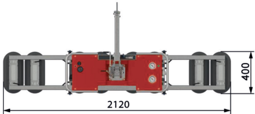
Erweitert 500 kg
